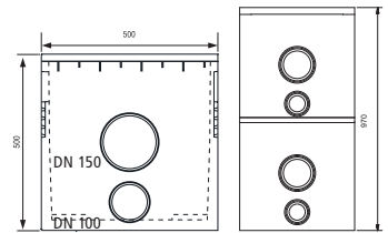
Zandvang/Afvoerput Verhoogde zandvang/afvoerput incl. verzinkte emmer
