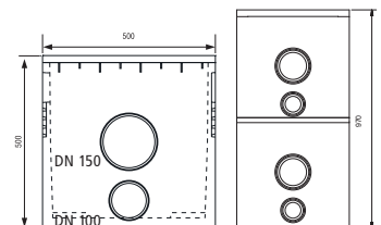
Zandvang/Afvoerput Verhoogde zandvang/ incl. verzinkte emmer afvoerput
