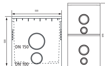
Zandvang/Afvoerput incl. verzinkte emmer Verhoogde zandvang/afvoerput
