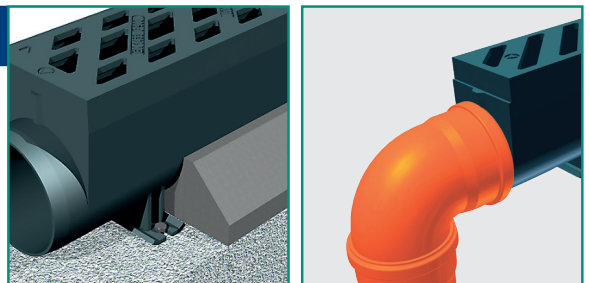
Verbindingen met standaard kunststofbuizen
