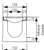
Gootelement 1000 mm bouwlengte
