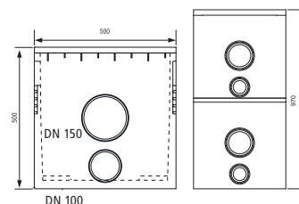
Zandvang/Afvoerput Verhoogde incl. verzinkte emmer zandvang/afvoerput
