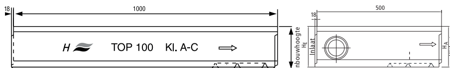
Goothelement 1000 mm bouw lengte
