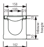
Gooitelement 1000 mm Lengte
