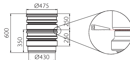
Tussenschacht DN400 incl. rubberafdichting. Kan op maat worden gezaagd.
